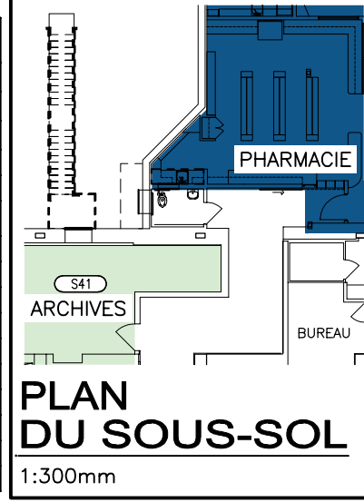
PLAN DU SOUS-SOL 1:300mm
