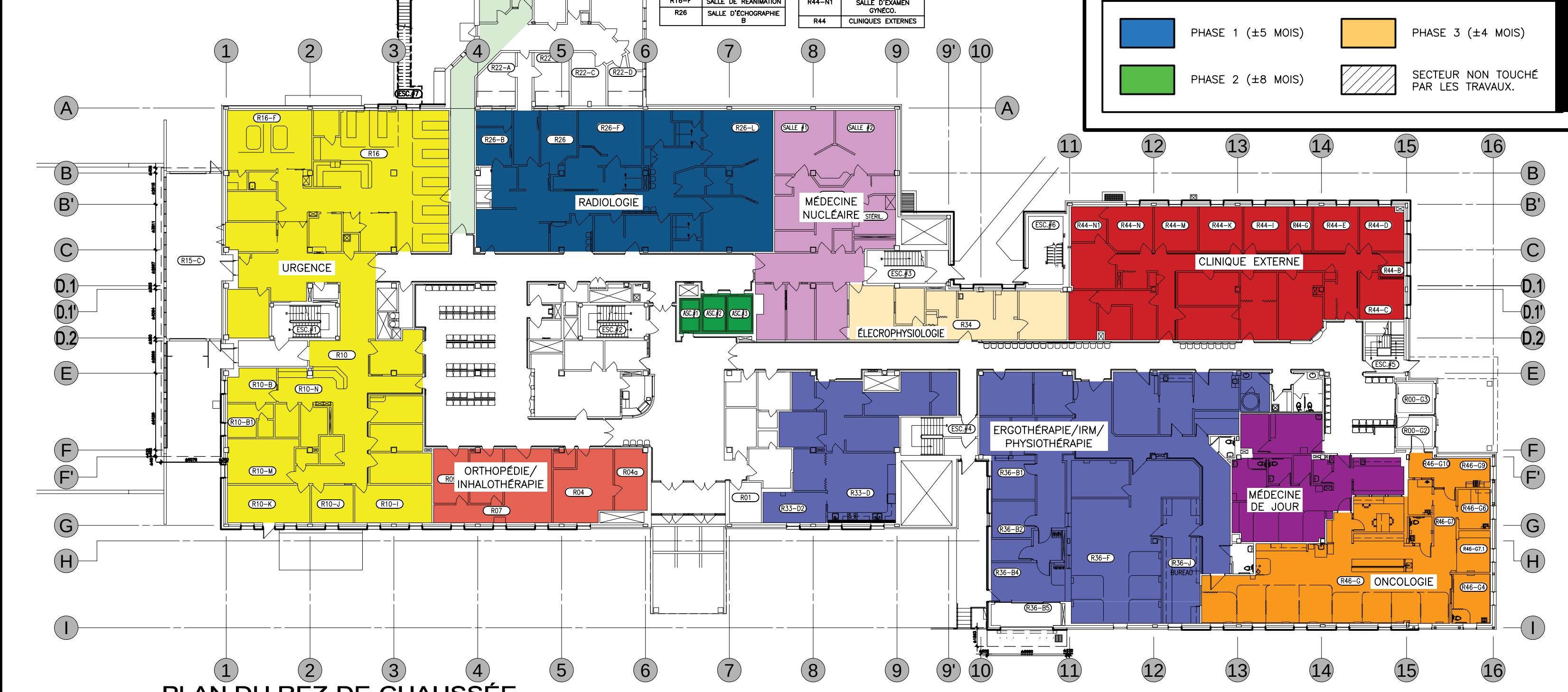
PLAN DU REZ-DE-CHAUSSEE 1:300mm
